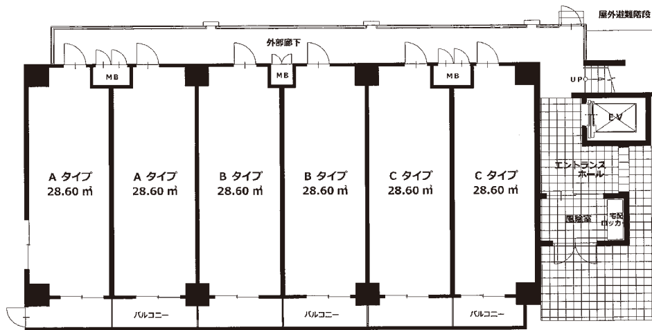
1階 平面図
