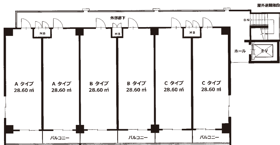
基準平面図
