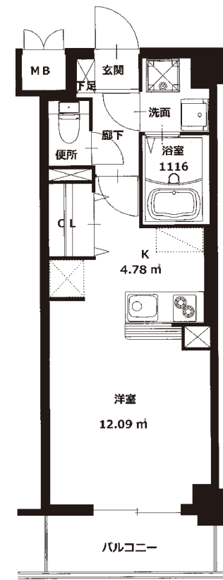
Bタイプ/28.60㎡
