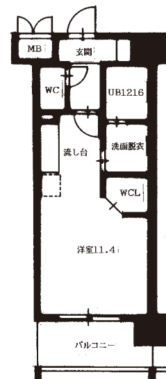
Cタイプ [28.22㎡]
