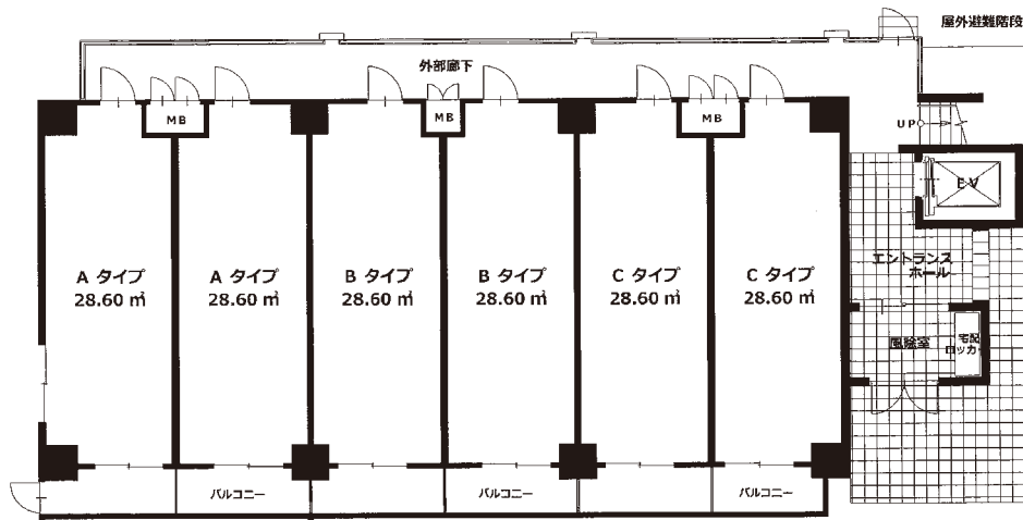
1階 平面図
